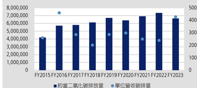
圖 12：碳排放量
